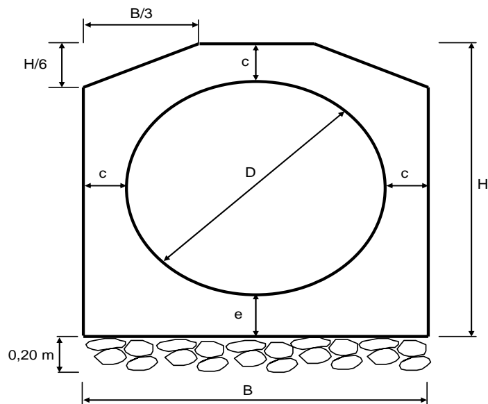
ESQUEMA TUBERIA FABRICADA EN SITIO
